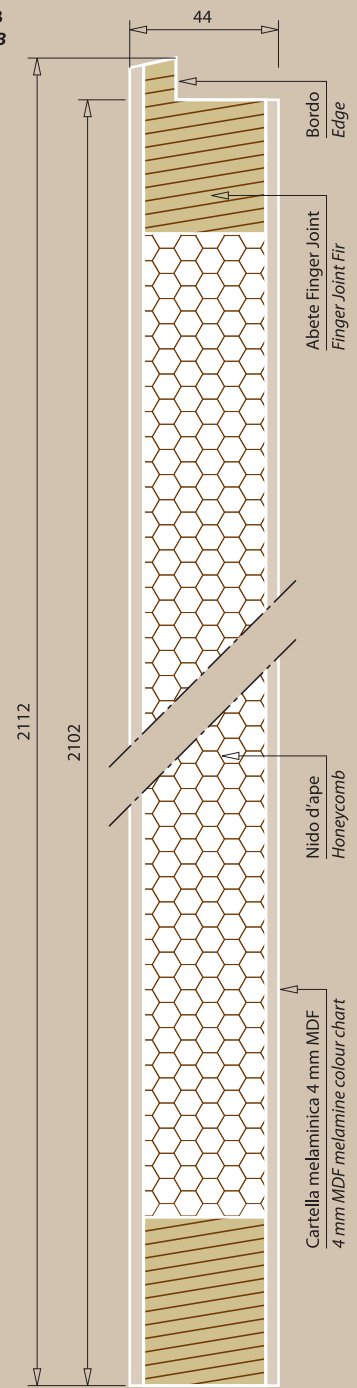
Sez. B - B Sect. B - B
